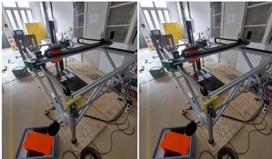
obr. 1.1 - Robotický manipulátor
